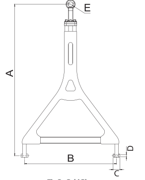
Tip 3 - Çeki Oku Type 3 - Drawbar Eye
